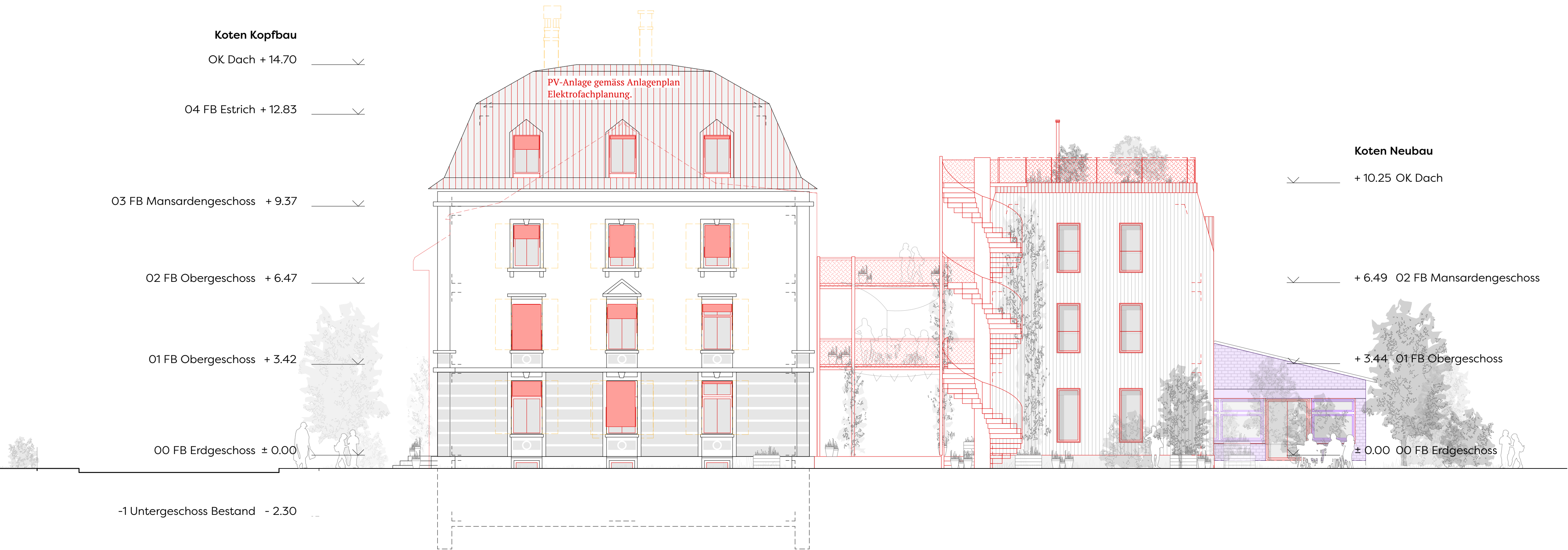
Ansicht Südost
